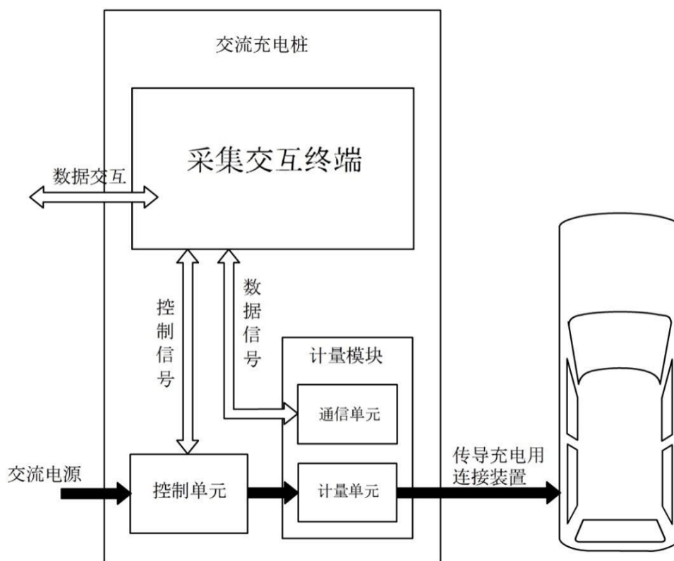
图 1 充电桩工作原理结构框图
